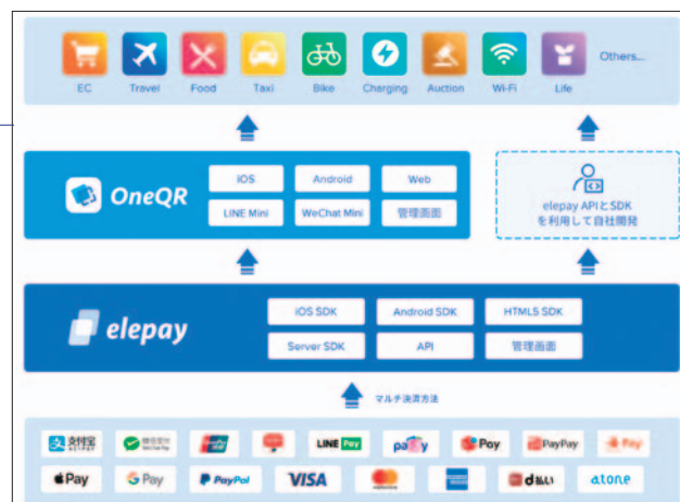
サービス、elepay/OneQR、決済手段の位置関係
